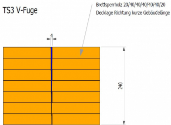
Schnitt V-Fuge
